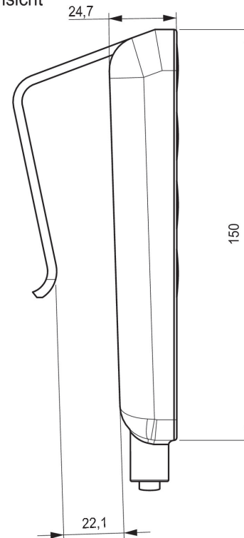
Seitenansicht
