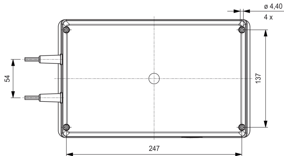
Draufsicht
